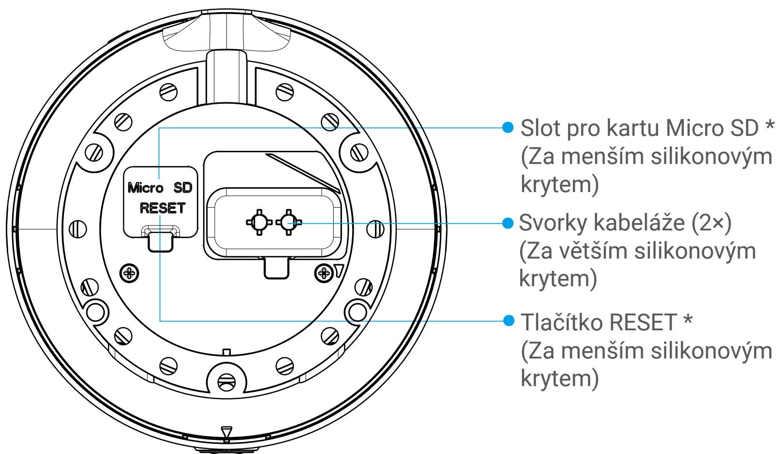
Spodní pohled
