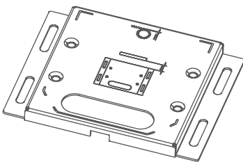
Montážní základna (1×)
